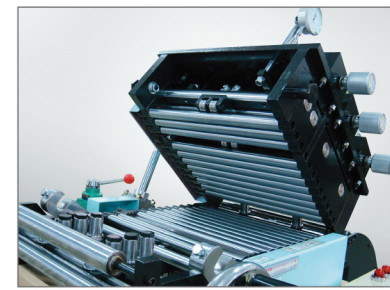
整平頭掀開裝置
