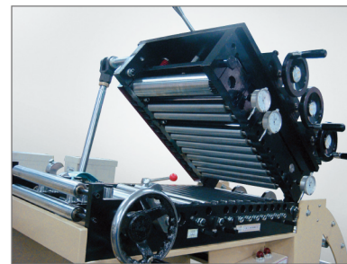
整平頭掀開裝置
