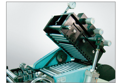
整平頭掀開裝置
