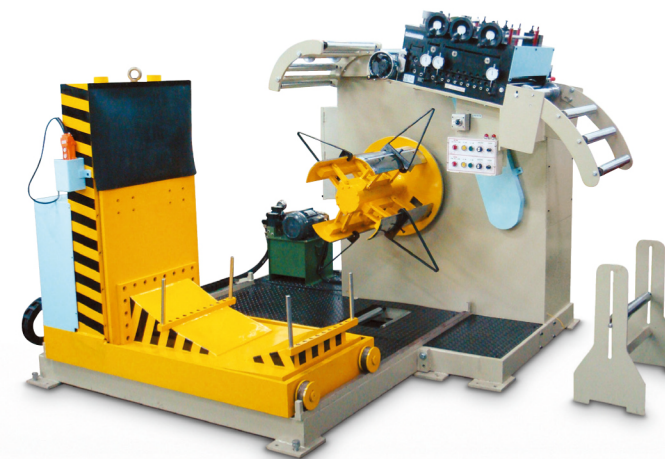
GMT / GWT / GXT / GOT / GLT 系列 入料台車/油壓擴張裝置
